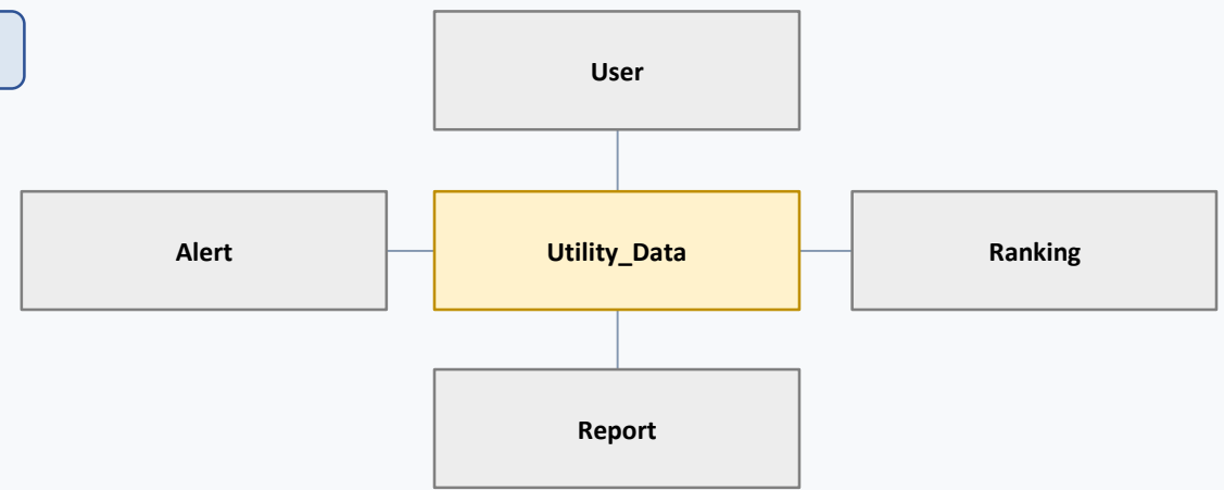
ER Diagram
